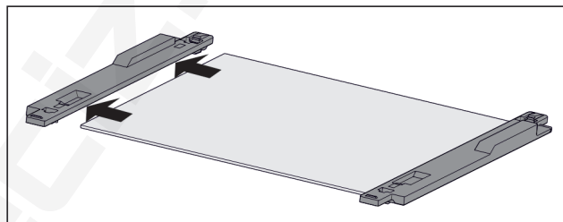
Fig. 45 Üveglap tartóelemekkel
