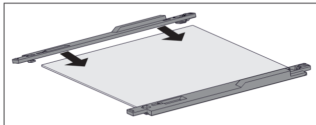
Fig. 46 Üveglap tartóelemekkel
